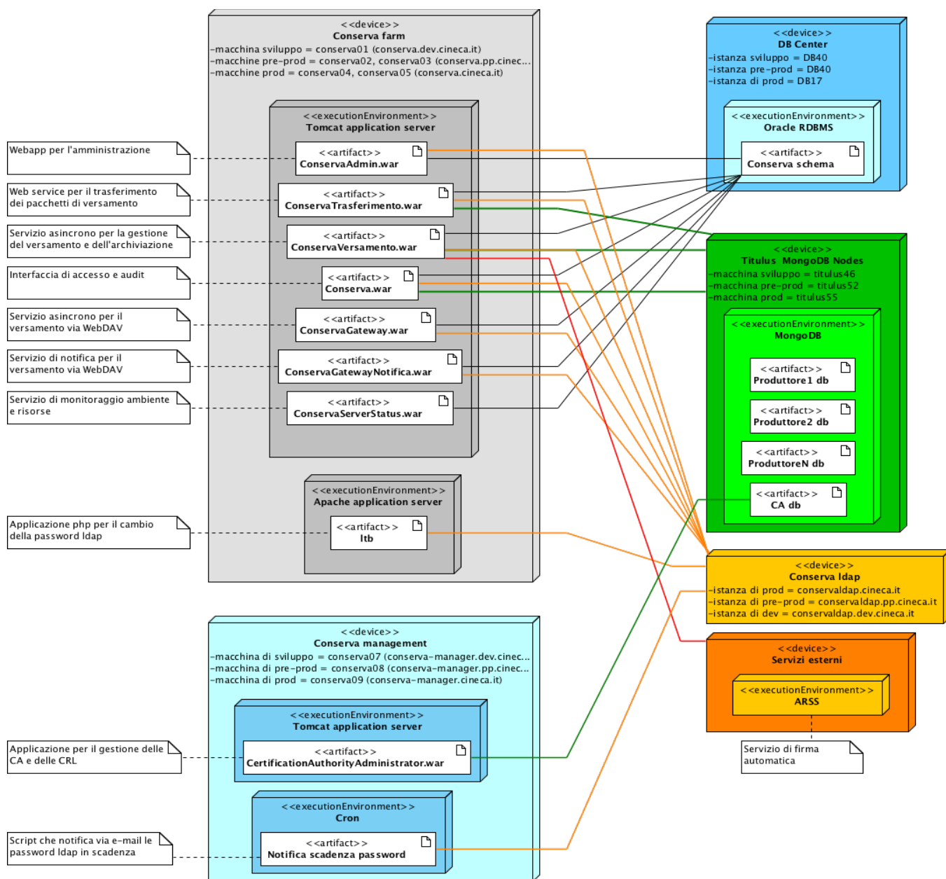
Figura 3 - Diagramma descrittivo dei componenti di Conserva
